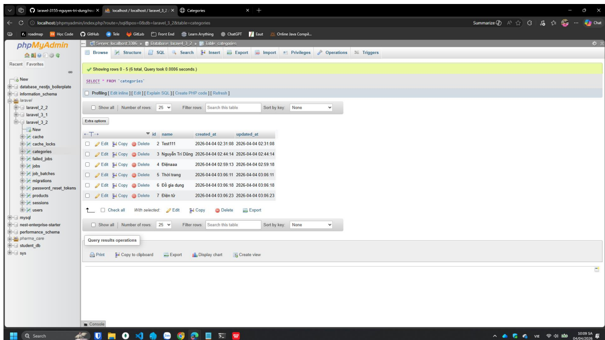
Hình 12: Database categories
