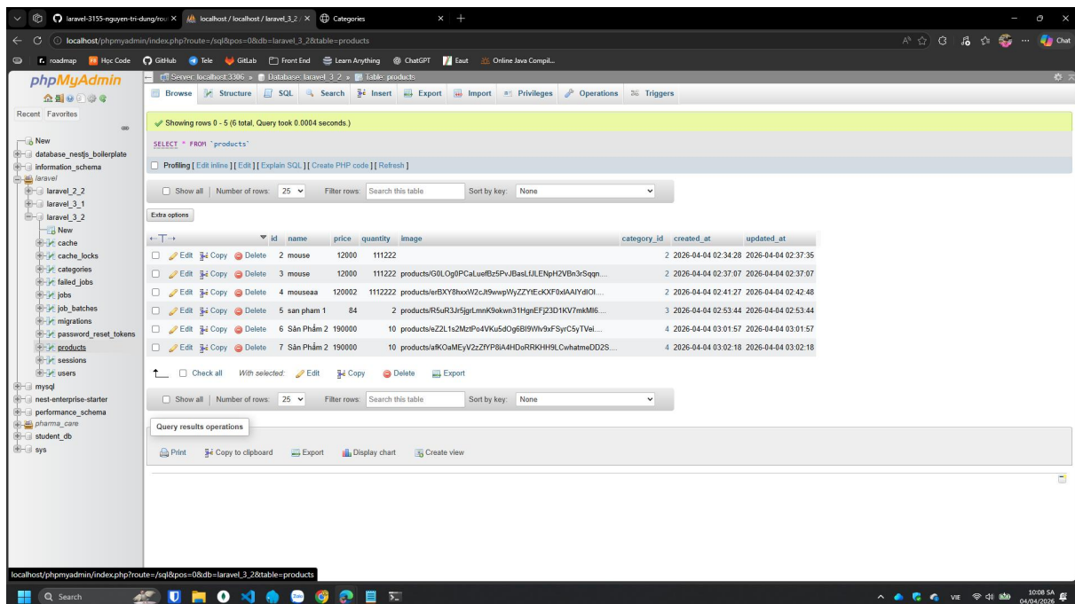
Hình 8: Database products
